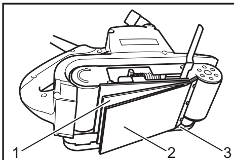
► 1. Plaque métallique 2. Plaque de carbone 3. Rondelle de courroie
