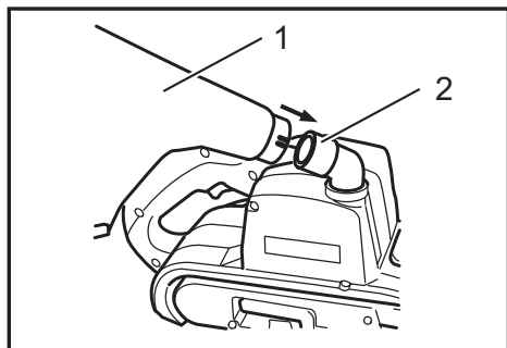
► 1. Sac à poussières 2. Buse d'éjection de la poussière
